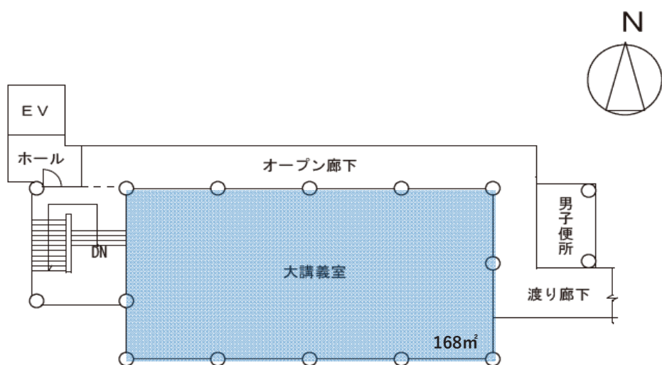
4号棟3階平面図 S = 1 / 400
