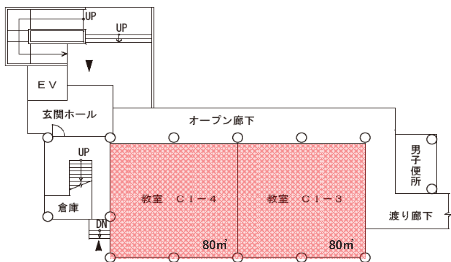
4号棟1階平面図 S = 1 / 400
