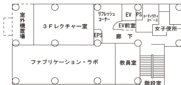
6号棟3階 平面図S=1/400
