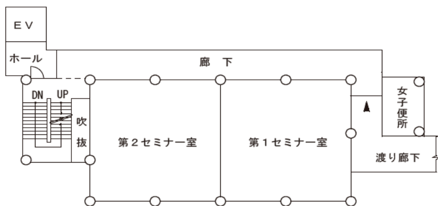
4号棟3階平面図 S = 1 / 400
