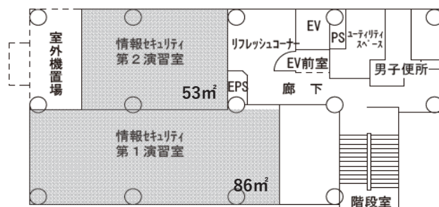
6号棟4階 平面図S=1/400
