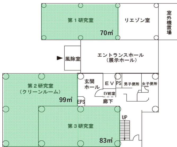
6号棟1階 平面図S=1/400
