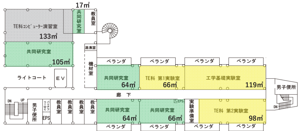
1号棟4階 平面図S=1/600
