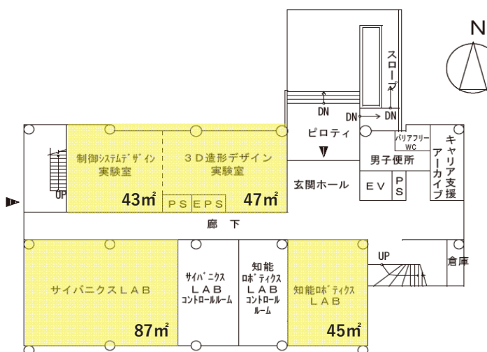
5号棟1階平面図 S = 1/400
