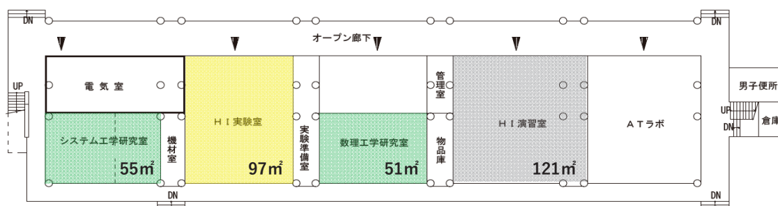
3号棟1階 平面図S=1/400
