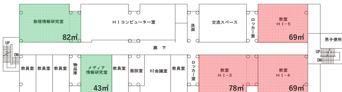
3号棟2階 平面図S=1/400
