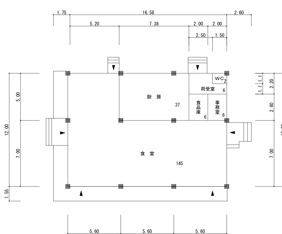
平面図 S=1/200 床面積 202 m 2
