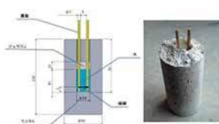
衝撃波パルスパワーの研究 Research for shockwave pulse power
