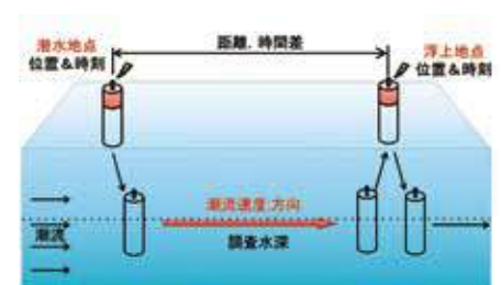
定水深浮遊体による潮流観測の研究 Research for tide observation using floating body
