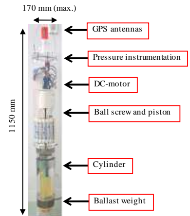
図 1 定水深フロートの全体図
