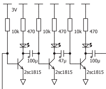
図26 信号機の回路図
