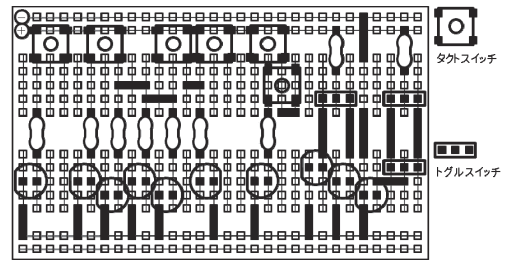
図9 スイッチ付きLED点灯回路の配線例
