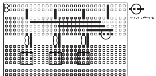
図11 光の三原色回路の配線例
