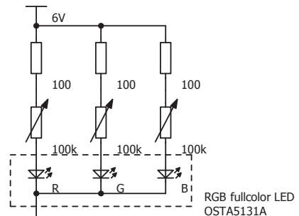
図10 光の三原色回路の回路図
