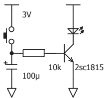
図12 シンプルタイマ回路の回路図
