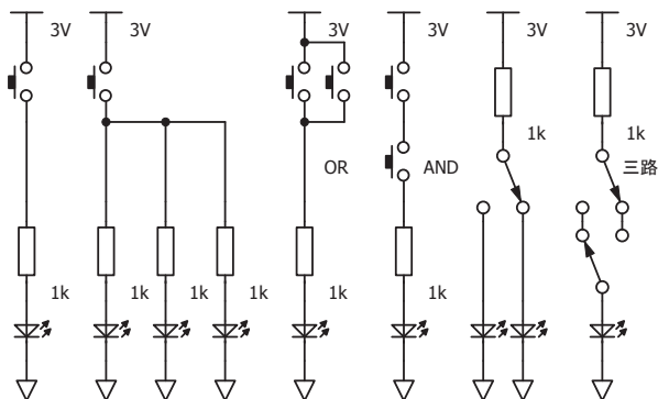
図8 スイッチ付きLED点灯回路の回路図
