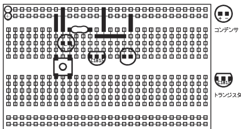
図13 シンプルタイマ回路の配線例
