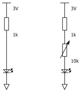
図6 LED点灯回路の回路図
