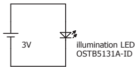
図2 イルミネーションの回路図
