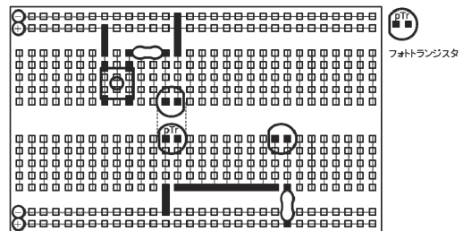
図23 シンプル光通信の配線例
